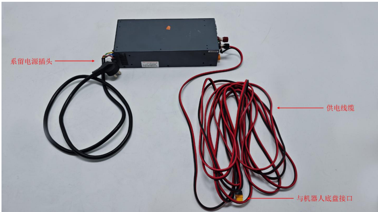
系留电源与供电线缆示意图
