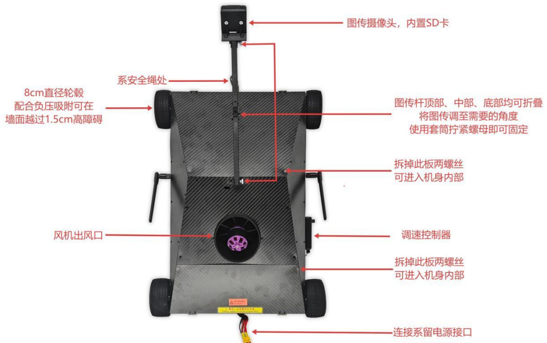
负压吸附爬壁机器人底盘部件示意图
